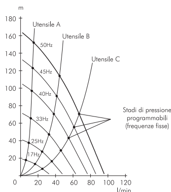
Fig. 6: Frequenze fisse
