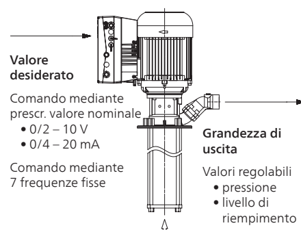
Fig. 4: Schema di un comando
