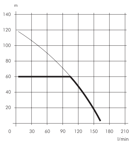
Fig. 3: Regolazione della pressione limitata a max 6 bar
