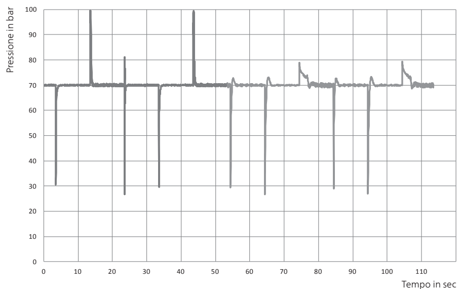
Valvola limitatrice di pressione standard Regolazione OFFSET attiva
