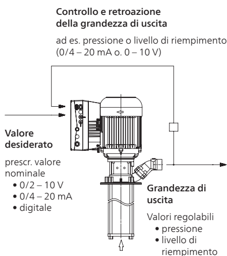
Fig. 2: Schema di una regolazione
