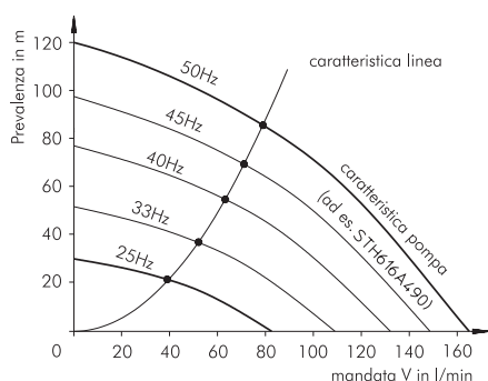
Fig. 1: Diagramma delle curve caratteristiche
