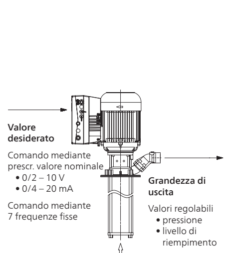
Fig. 4: Schema di un comando
