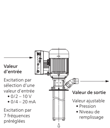
Fig. 4 : Schéma d'un pilotage
