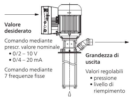
Fig. 4: Schema di un comando
