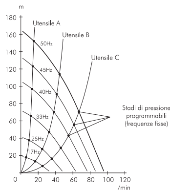
Fig. 5: Frequenze fisse
