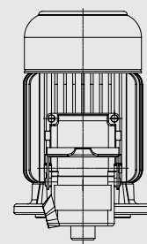
Connettore a spina in basso Non realizzabile per tutti i modelli in relazione all'altezza del motore.
