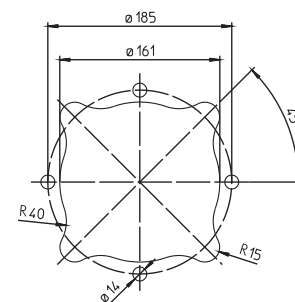
Blechausschnitte TFS3 / TFS4
