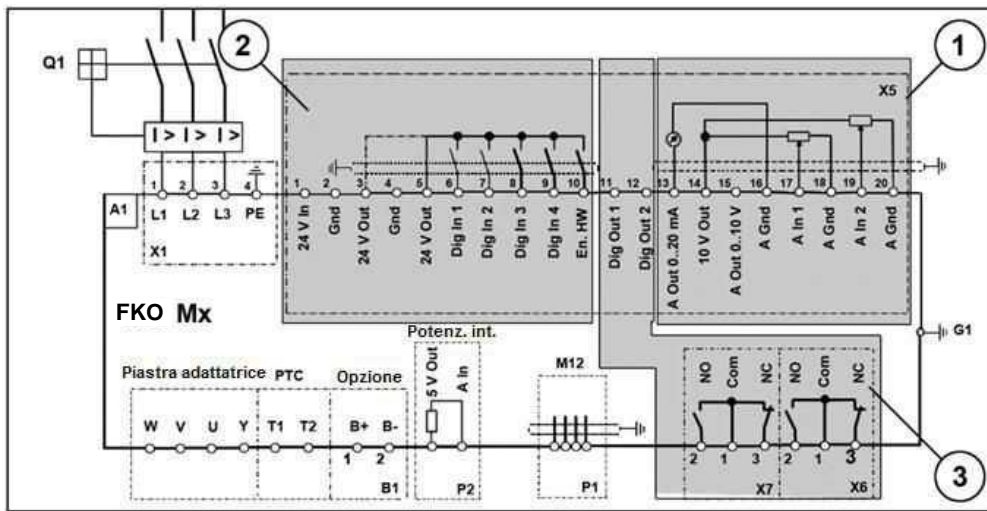
Fig. 14: Connessioni di comando
