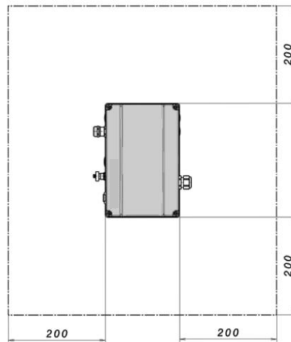
Fig. 15: Distanze minime
